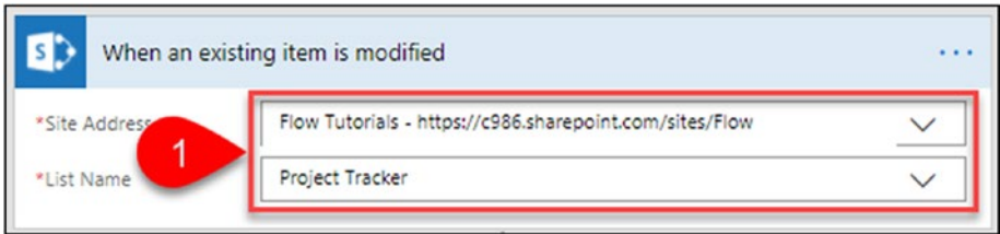
Figure 2-28. Trigger parameters
