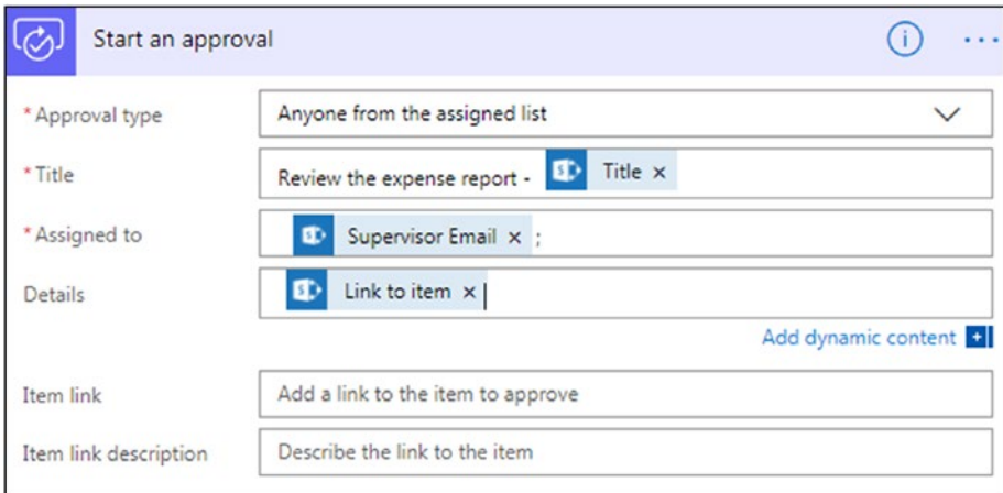
Figure 3-33. Add parameters
