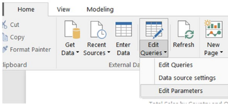
Figure 13-6. Editing parameters
